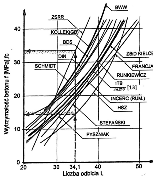
Rys. 1. Przykładowe zależności empiryczne f_c - L dla sklerometrów (młotków) Schmidta typu N, przyjęte w Polsce i innych krajach [5]
